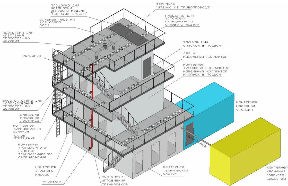
Рис.1 Автоматизированный учебно-тренировочный огневой комплекс
